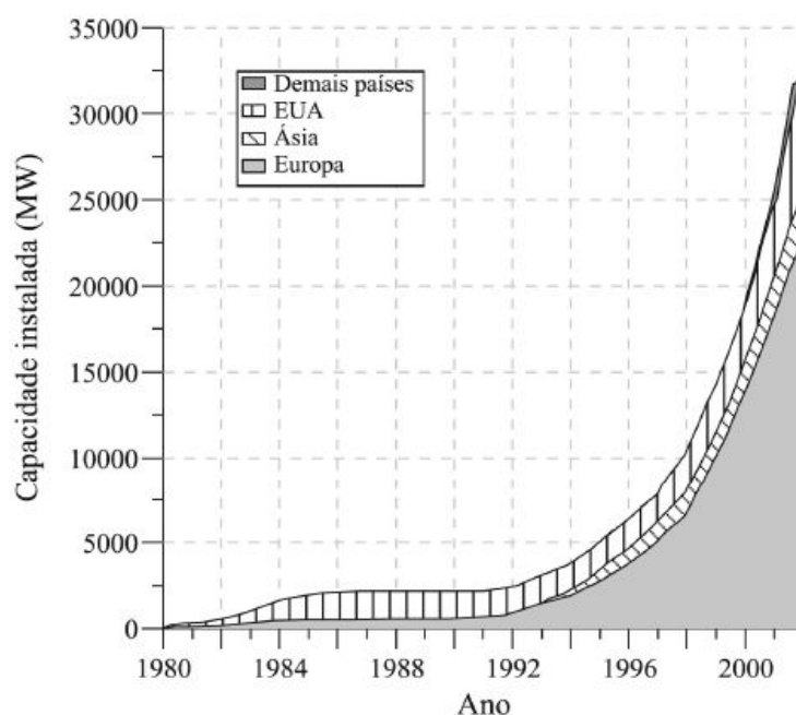
Figura 3.2 – Evolução da capacidade instalada de geração eólica de eletricidade no mundo. Fonte: R. Gasch and J. Twele, 2002.
