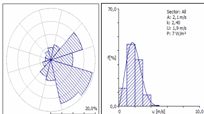
Figura 9.4 – Distribuição estatística dos ventos a 10m de altura coletados a partir do dia 14/02/2009 no Observatório Espacial do Sul.
