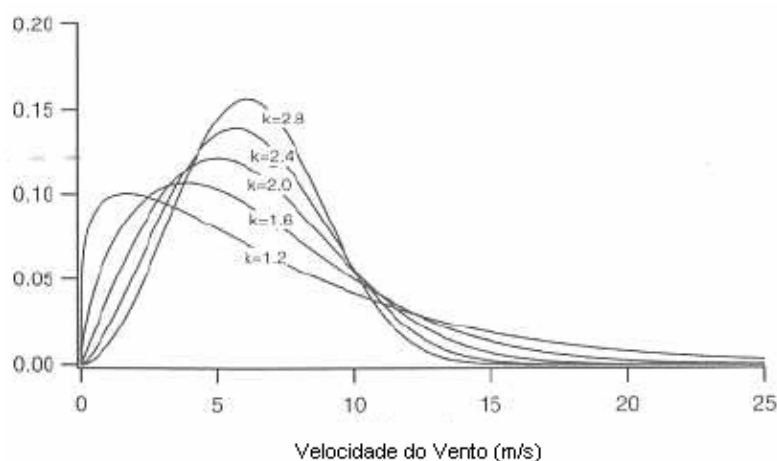
Figura 6.3 – Distribuição de Weibull para diferentes fatores de forma. Fonte: Manwell, et al., 2002.
