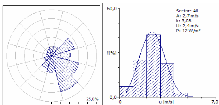
Figura 9.5 – Distribuição estatística dos ventos a 25m de altura coletados a partir do dia 14/02/2009 no Observatório Espacial do Sul.
