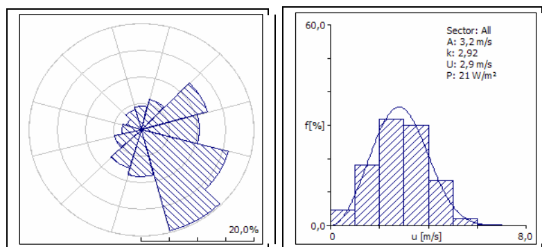
Figura 9.6 – Distribuição estatística dos ventos a 50m de altura coletados a partir do dia 14/02/2009 no Observatório Espacial do Sul.
