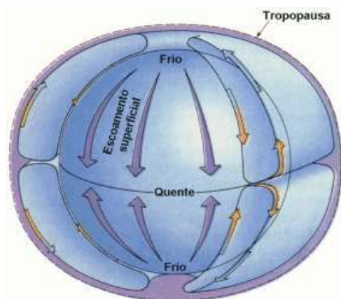
Figura 4.8 – Circulação global numa Terra sem rotação (Hadley). Fonte: Meteorologia Básica – Notas de Aula (2009).
