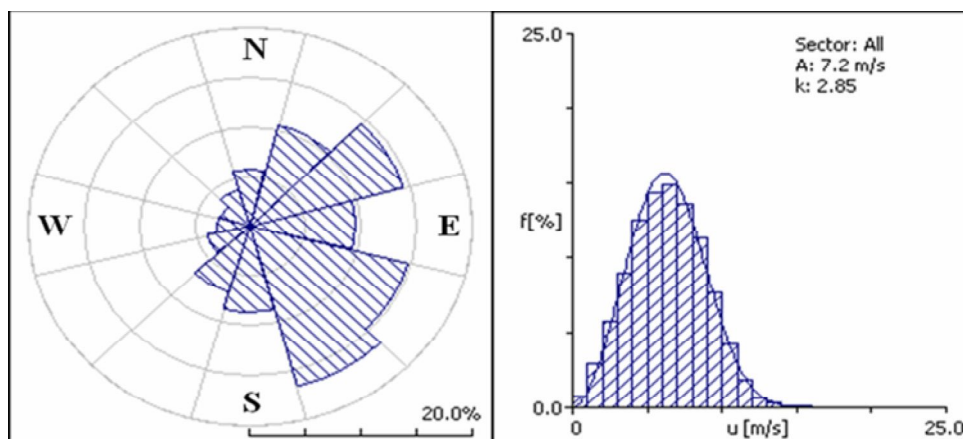
Figura 9.3 – Distribuição estatística dos ventos a 50m de altura medida no Observatório Espacial do Sul – OES/CRS/INPE - MCT.
